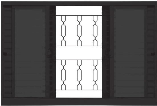
VENEZIANA 6 FOLHAS 2 FIXAS GR. ELO.
